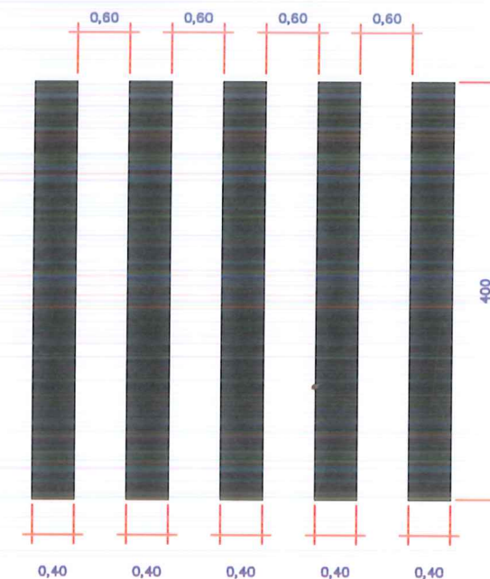
DETALHE DA FAIXA PARA PEDESTRES SEM ESCALA
