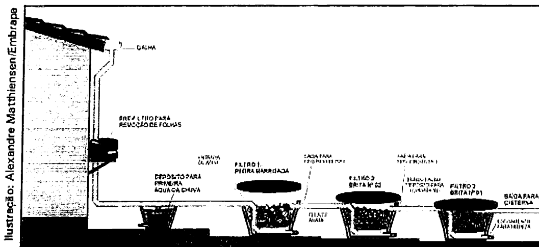
Figura 31 – Resumo do sistema de filtragem.
