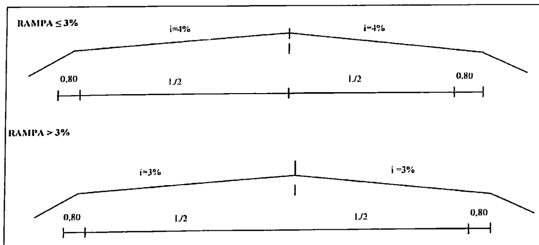
Figura 8: Inclinação transversal
