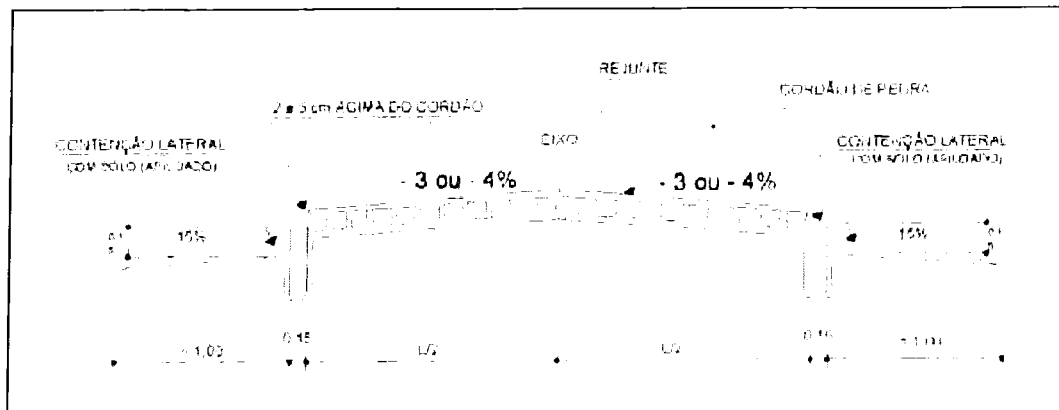
Figura 13 – Assentamento das Pedras
