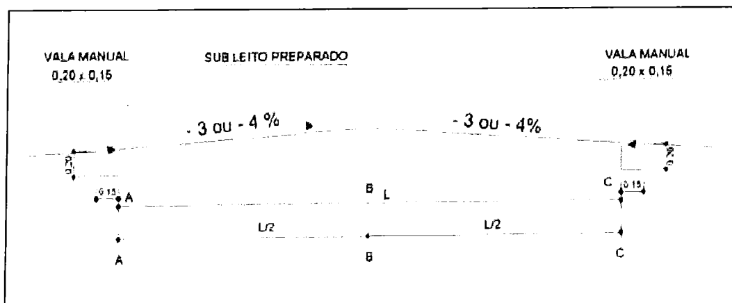
Figura 9 – Valas Laterais
