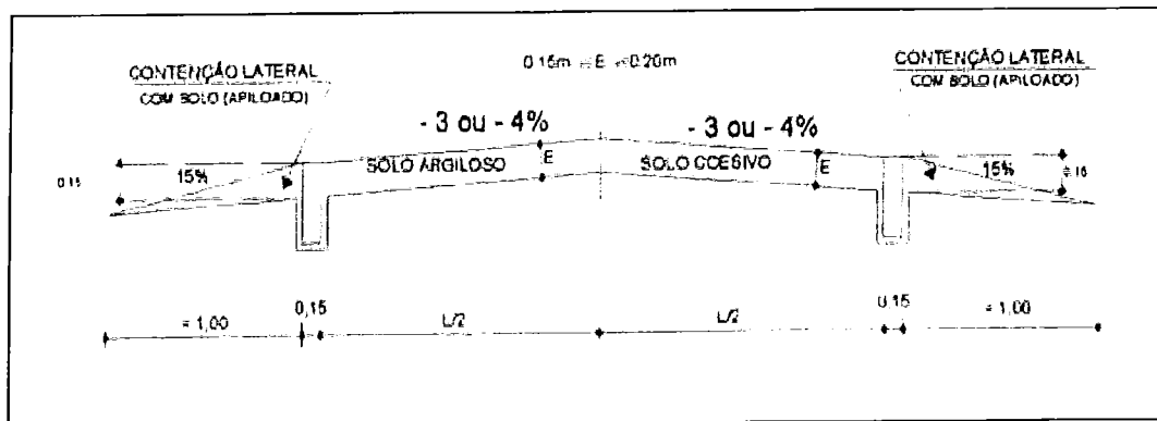
Figura 12 – Colchão de Solo
