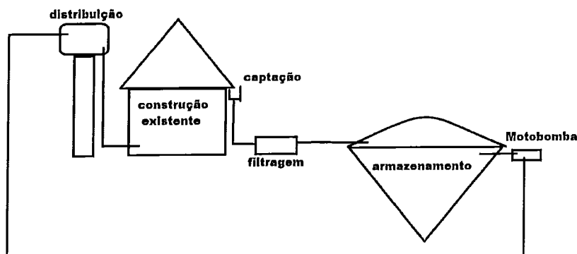
Figura 21 – esquema básico do sistema proposto.
