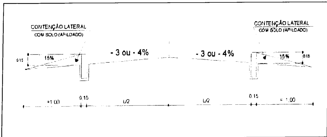
Figura 11 – Contenção Lateral
