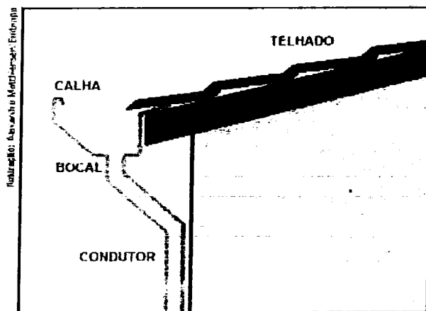
Figura 24 – Instalação das Calhas e Condutores de Descida.
