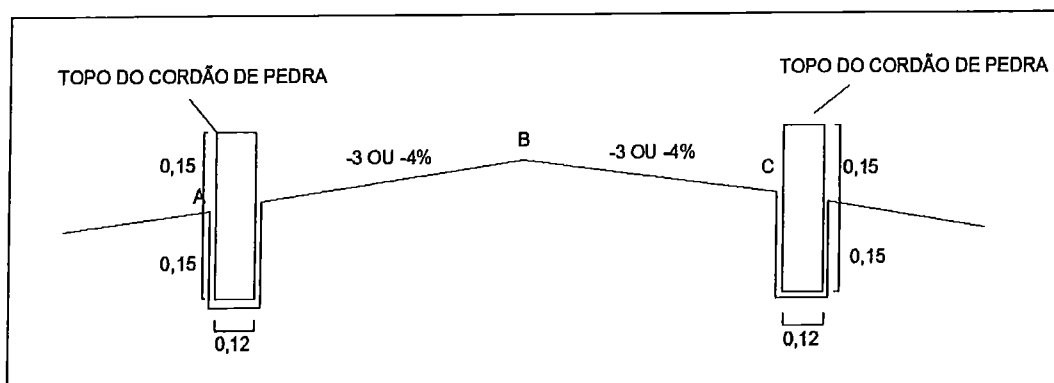
Figura 10 – Cordão Lateral de Pedra
