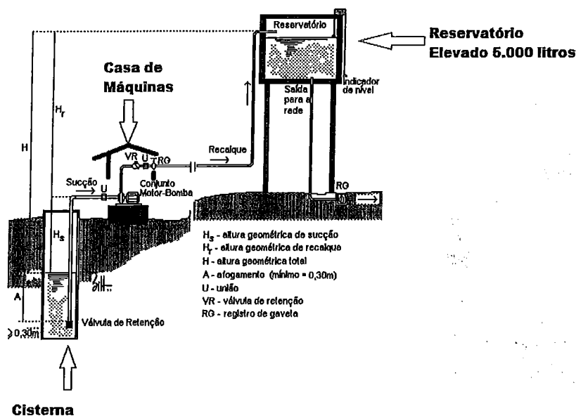
Figura 32 – Sistema de Distribuição Resumido
