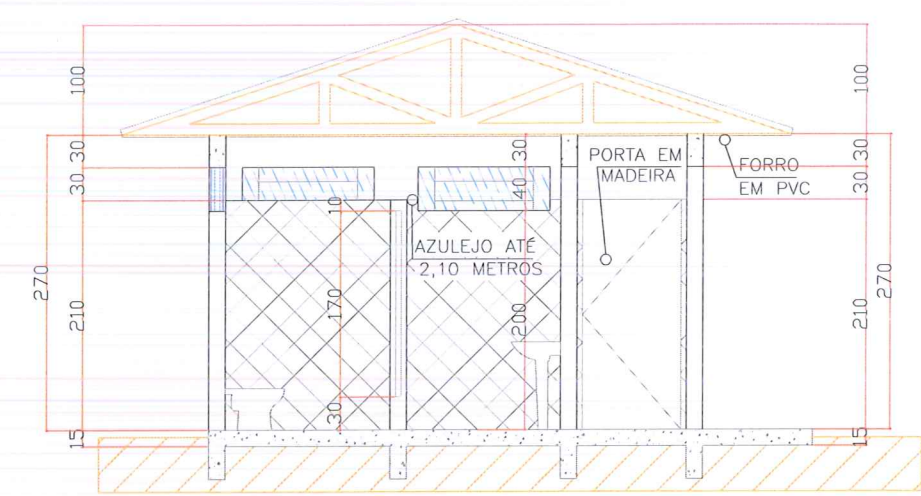
CORTE BB
