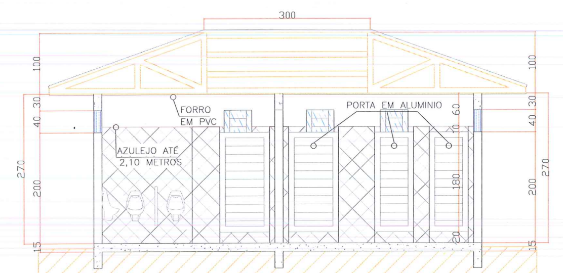
CORTE AA
