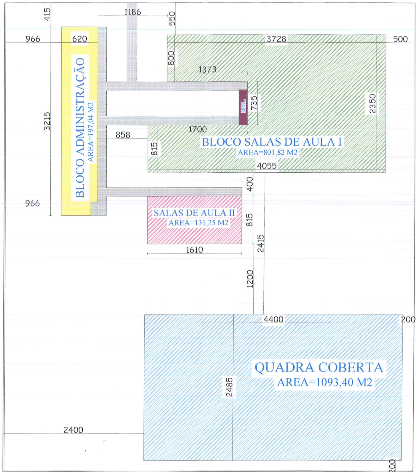
PLANTA DE IMPLANTAÇÃO ESCALA: 1/250
